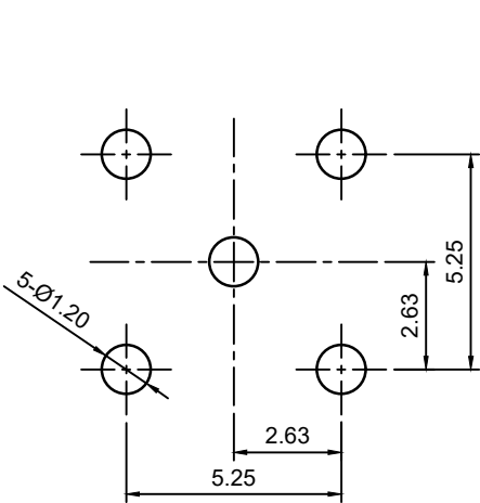
推荐PCB安装孔位
